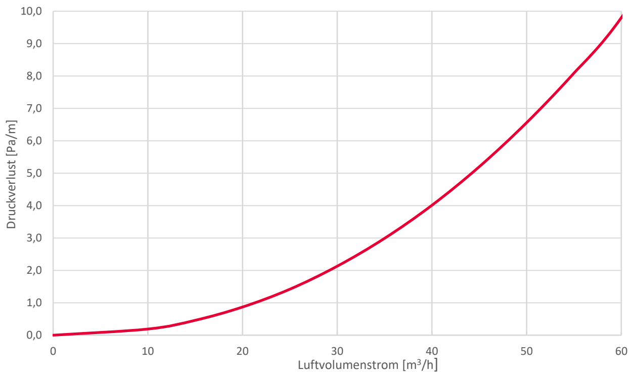
Druckverlust - Rohr 75 HEATPEX ARIA
